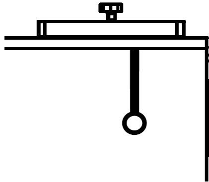
Abbildung 7: Kurzschlussklappenhebel in geschlossener Stellung.
