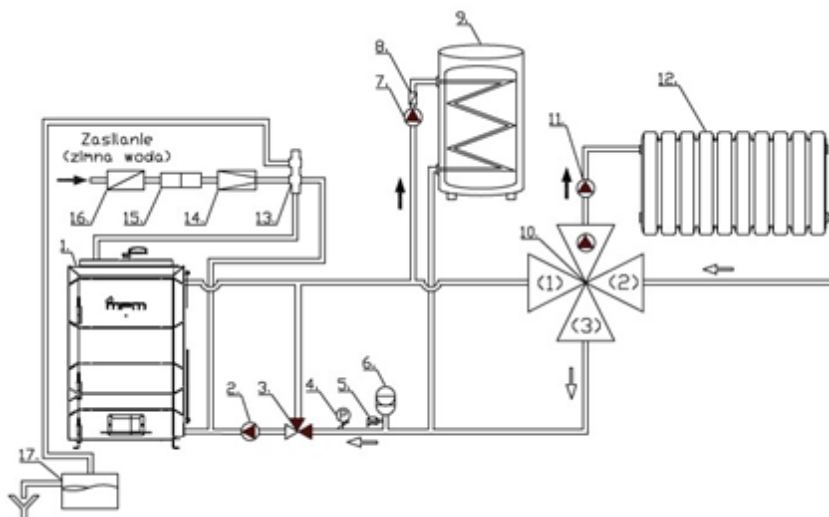
Abbildung 4: Beispielschema für den Anschluss des MPM Wood Plus Holzessels in einem geschlossenen System.
