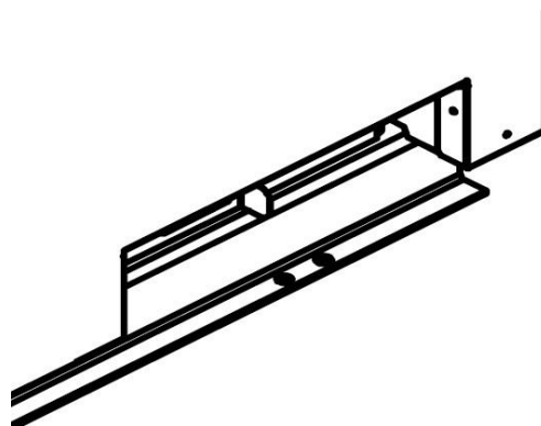
Abbildung 8: Lage der Klappen für die Sekundärluftzufuhr
