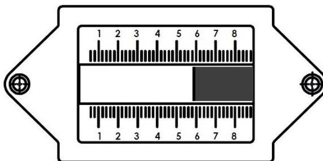
Abbildung 10: Einstellung der Sekundärluftmenge
