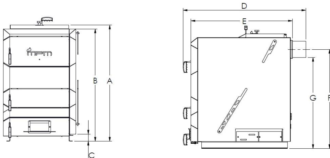
Abbildung 2: Grundlegende Abmessungen des MPM Wood Plus Holzkessels
