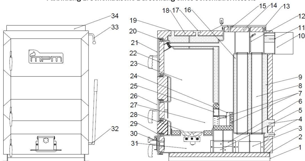
Abbildung 1: Schematische Darstellung eines Seitenladerkessels
