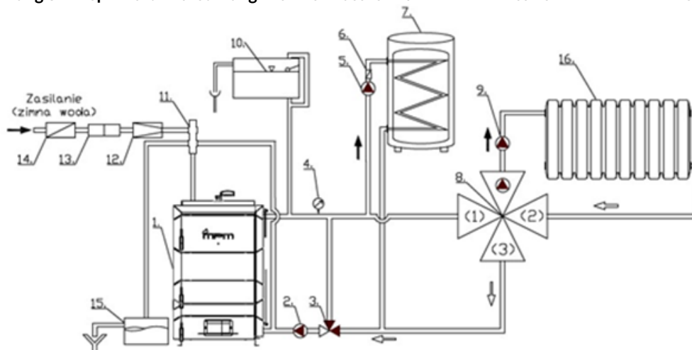
Abbildung 3: Beispielhafte Darstellung des Anschlusses des MPM Holzessels in einem offenen System.
