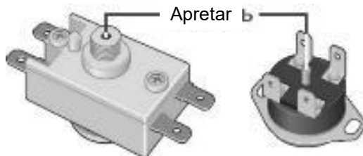
Figura 3. Posición de botón del interruptor térmico
