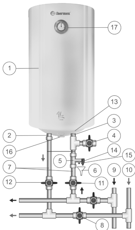
Paveikslas 1. EVŠ prijungimo prie vandentiekio schema
