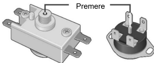
Fig. 3. Schema di posizionamento del gambo dell'interruttore termico
