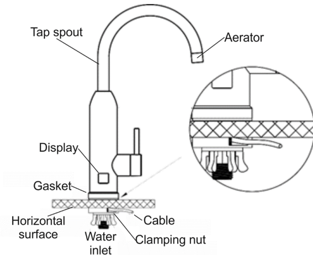
Abb. 2. Installation mit dem Ausgang des Netzkabels unter der Spüle
