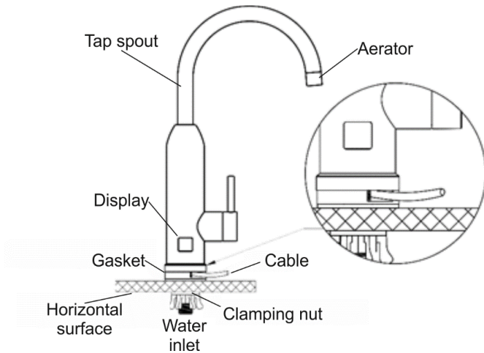
Abb. 1. Installation mit dem Ausgang des Netzkabels über der Spüle
