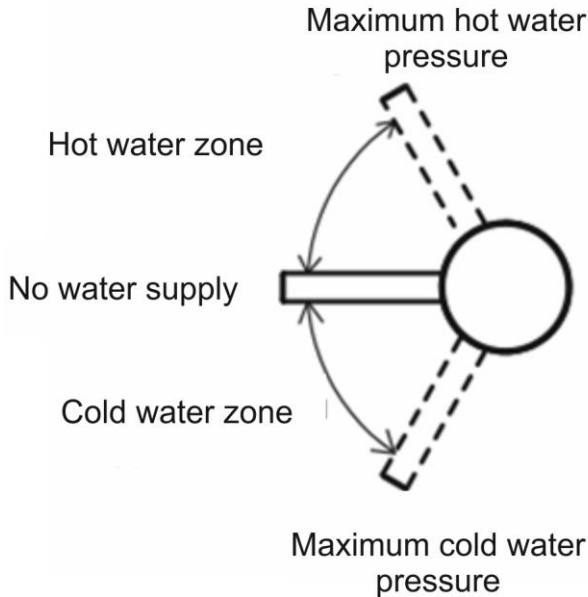
Abb. 3 Regelung des maximalen Wasserdurchflusses.
